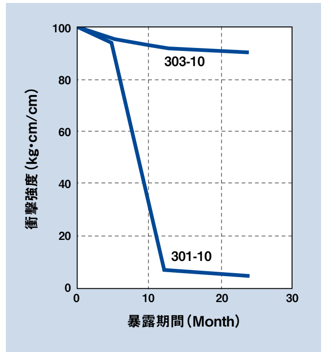
衝撃強度の変化 (条件 23°C)
