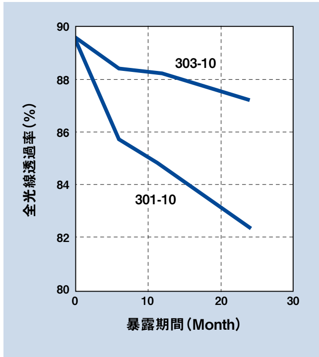
全光線透過率の変化
