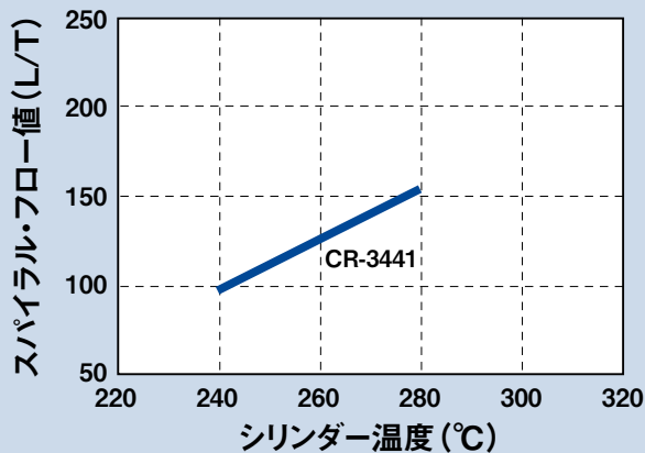
PC/PBTアロイ
